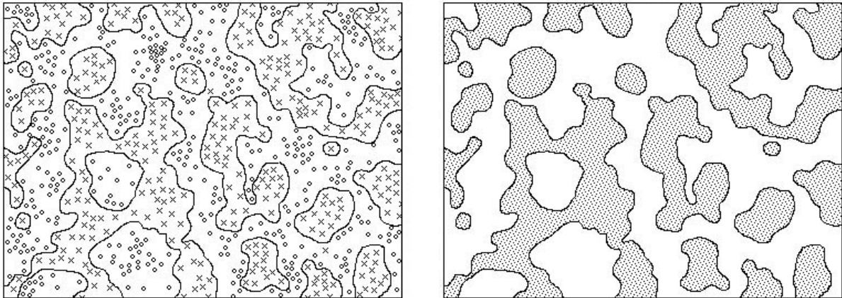
Phénomène de percolation
