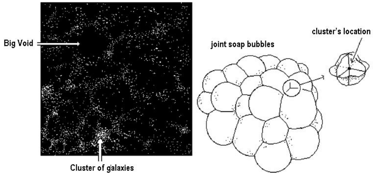
Structuration de la matière en bulles de savons jointives
